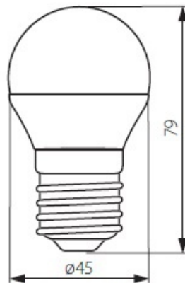
BIL0 6,5W T SMD E27
