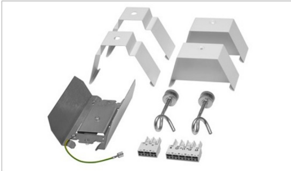
Zestaw zamykający (150340)
