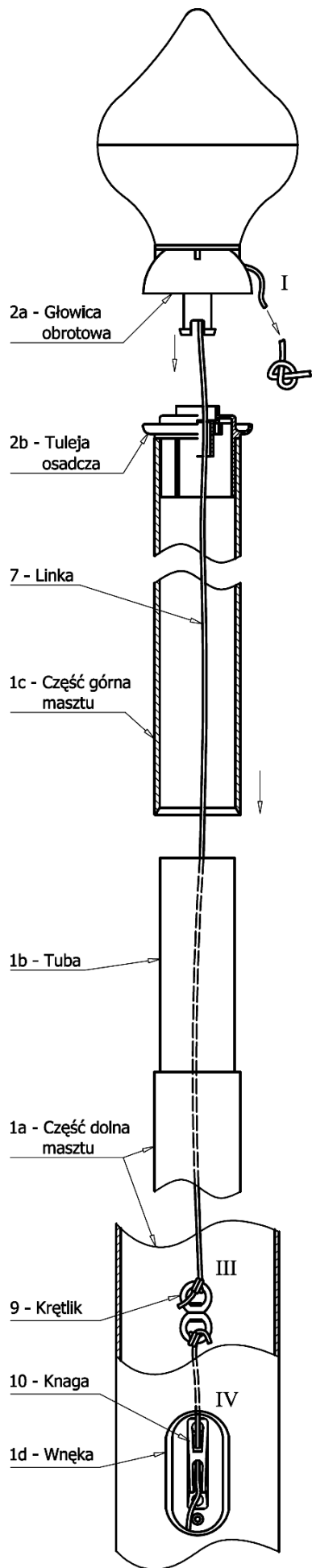
Rys.2. Schemat ułożenia linki w maszcie
