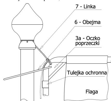
Rys.3. Schemat mocowania poprzeczki
