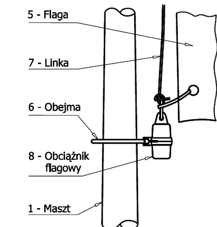
Rys.4. Schemat mocowania obciążnika
